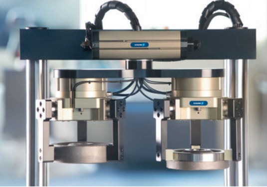
Schwenkeinheiten
